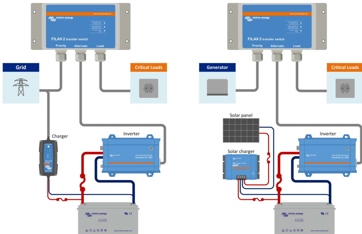
System Filax se záložním měničem/nabíječkou:
